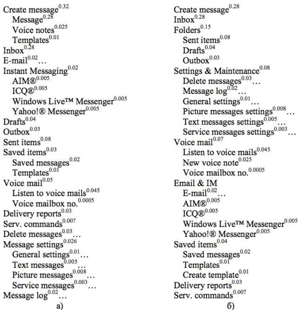
Рис. 4. Оригинальная и оптимизированная структура меню мобильного телефона
