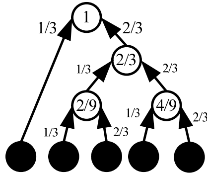
Рис. 3. Пример однородного дерева
