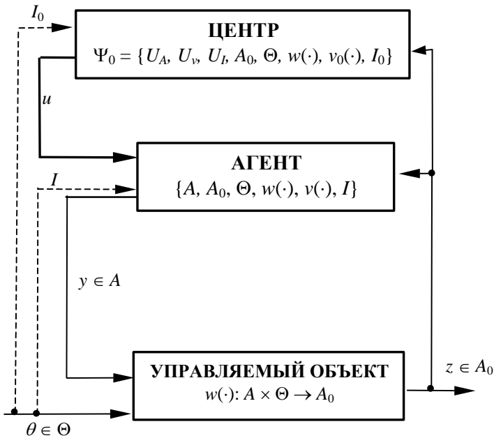
Рис. 2. Структура системы управления.
