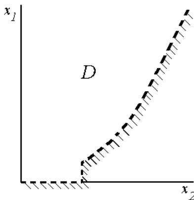
Рис. 10. Множество достижимости
